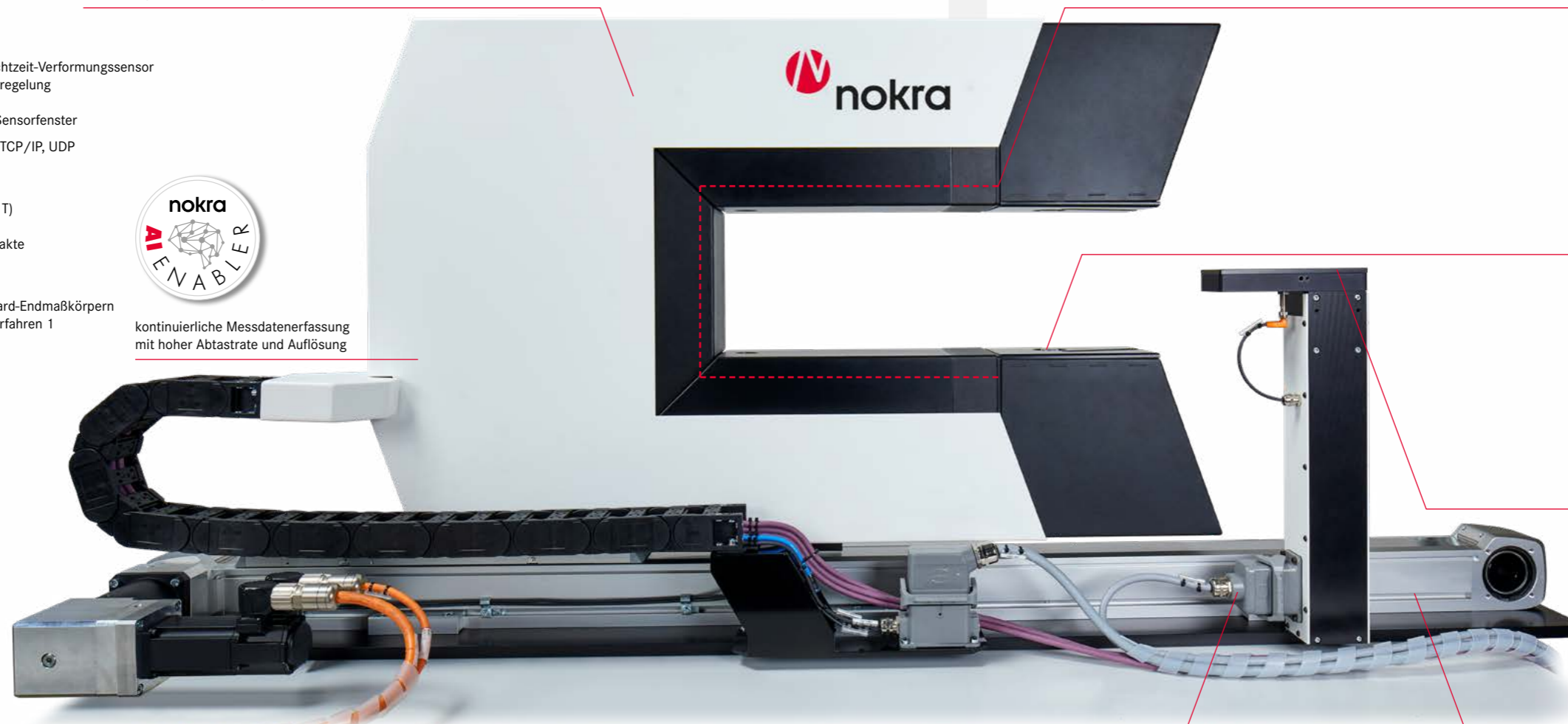
Ausführungen Messtiefe C-Bügel 500 / 1000 / 1500 / 2100 mm
